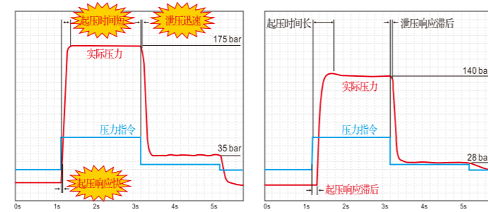
SPEED 168 动作响应快控制准确 竞争品牌160吨 动作响应慢，压力控制差
