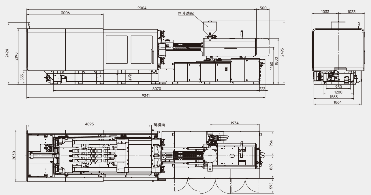
外形尺寸 (长×宽×高)
