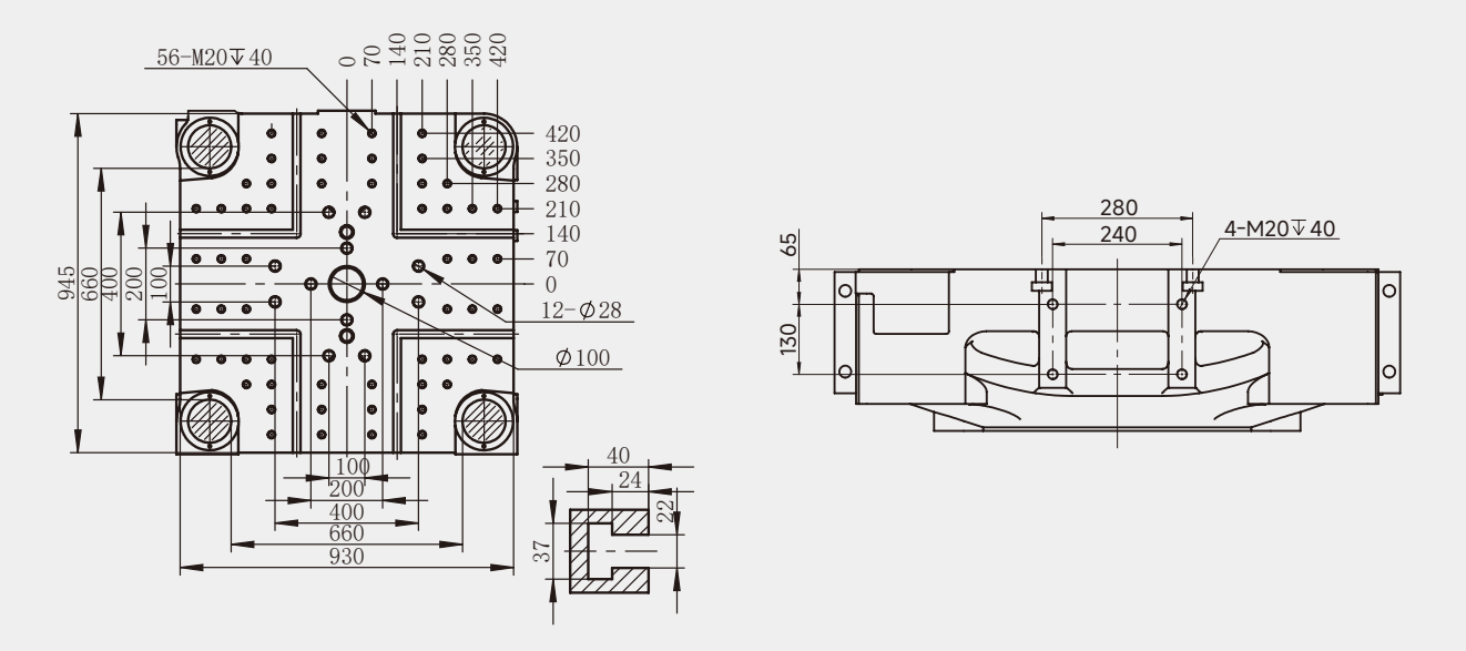
模板尺寸+机械手安装图
